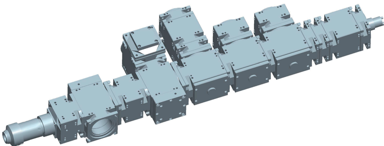
图15 光纤激光器光学参数测量仪分光器外观
